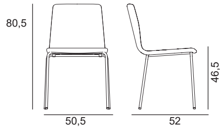
INGA 5683 L.50,5 x P.52 x H.80,5 cm, hauteur d'assise 46,5 cm
