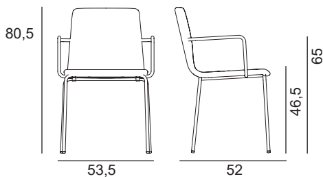
INGA 5684 L.53,5 x P.52 x H.80,5 cm, hauteur d'assise 46,5 cm
