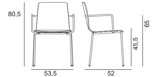
INGA 5664 L.53,5 x P.52 x H.80,5 cm, hauteur d'assise 45,5 cm
