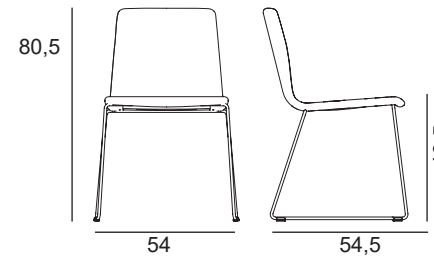
INGA 5689 L.54 x P.54,5 x H.80,5 cm, hauteur d'assise 46,5 cm
