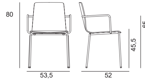
INGA 5614 L.53,5 x P.52 x H.80 cm, hauteur d'assise 45,5 cm
