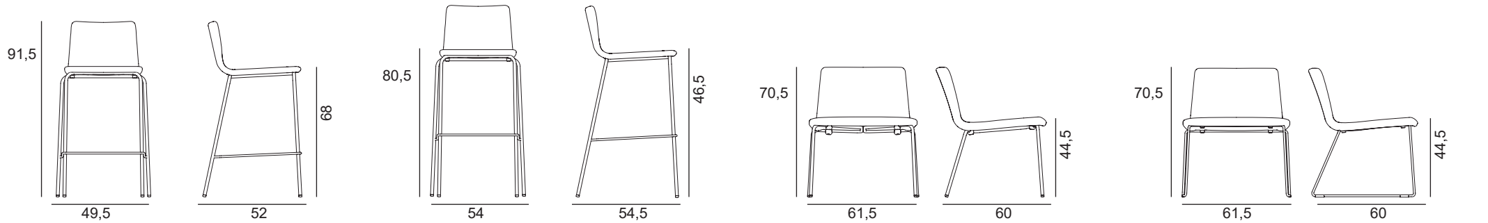
INGA 5686 L.49,5 x P.52 x H.91,5 cm, hauteur d'assise 68 cm | INGA 5687 L.50,5 x P.54,5 x H.101 cm, hauteur d'assise 78 cm | INGA 5681 L.61,5 x P.60 x H.70,5 cm, hauteur d'assise 44,5 cm | INGA 5688 L.61,5 x P.60 x H.70,5 cm, hauteur d'assise 44,5 cm
