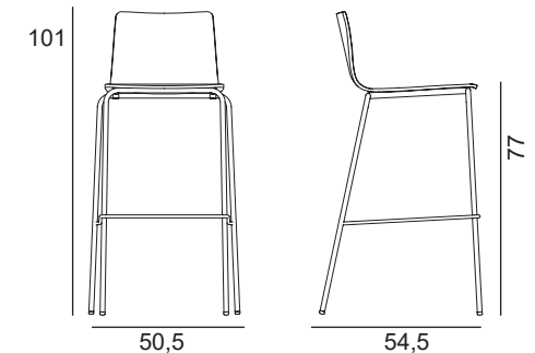
INGA 5617 L.50,5 x P.54,5 x H.101 cm, hauteur d'assise 77 cm
