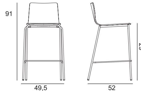
INGA 5616 L.49,5 x P.52 x H.91 cm, hauteur d'assise 67 cm
