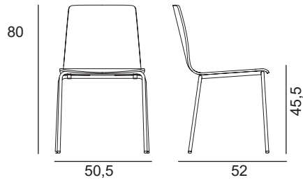
INGA 5613 L.50,5 x P.52 x H.80 cm, hauteur d'assise 45,5 cm
