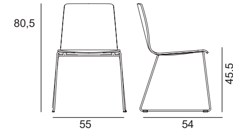
INGA 5669 L.55 x P.54 x H.80,5 cm, hauteur d'assise 45,5 cm
