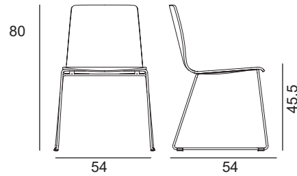
INGA 5619 L.54 x P.54 x H.80 cm, hauteur d'assise 45,5 cm
