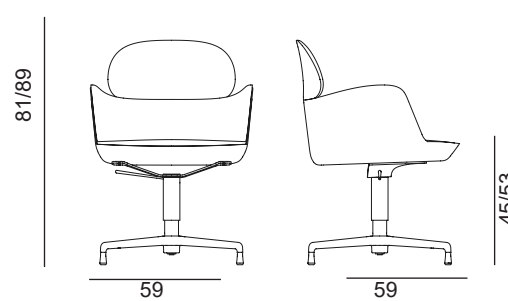
Fauteuil pivotant Ester 695 F, réglable en hauteur
