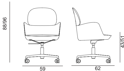
Fauteuil pivotant Ester 696, réglable en hauteur
