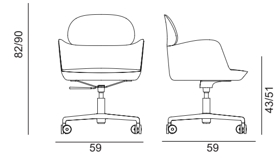
Fauteuil pivotant Ester 695, réglable en hauteur
