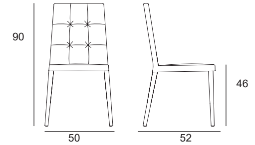
DRESS 533 L.50 x P.52 x H.90 cm, hauteur d'assise 46 cm
