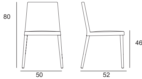
DRESS 530 L.50 x P.52 x H.80 cm, hauteur d'assise 46 cm
