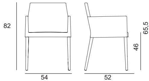
DRESS 535 L.54 x P.52 x H.82 cm, hauteur d'assise 46 cm
