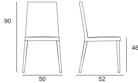
DRESS 531 L.50 x P.52 x H.90 cm, hauteur d'assise 46 cm
