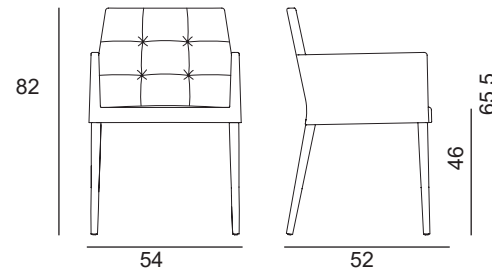
DRESS 536 L.54 x P.52 x H.82 cm, hauteur d'assise 46 cm
