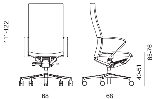
CIE 98 - chaise pivotante
