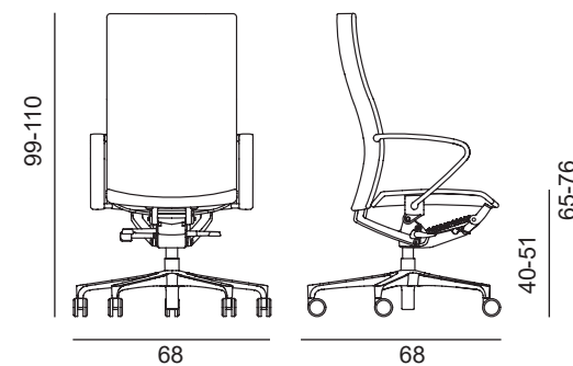
CIE 97 - chaise pivotante
