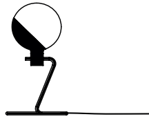
Lampe de table haute: base Ø 25 + H.57 cm
