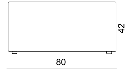
Pouf rond Ø 80 x H.42 cm
