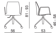
Chaise sur roulettes avec accoudoirs
